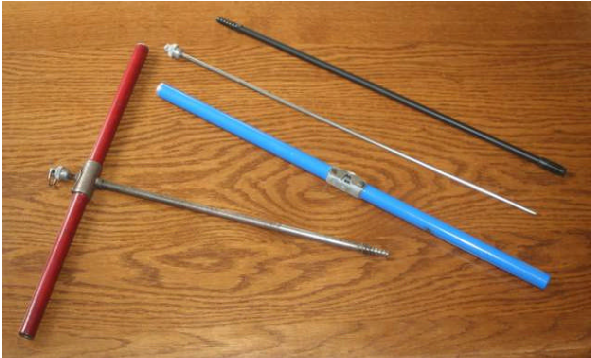
Figure 3 : Tarière de PRESSLER :
