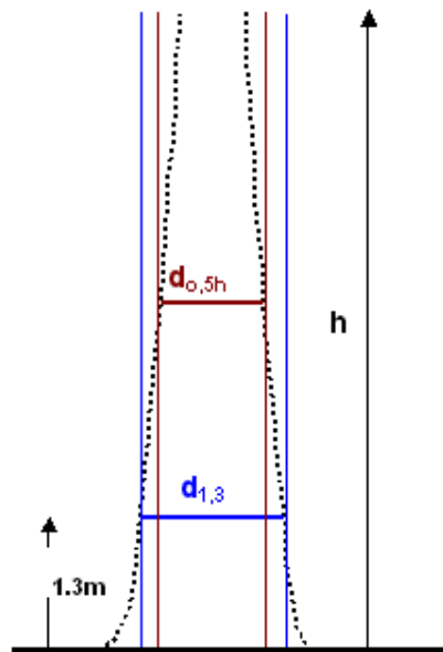
Figure 2 : Volume commercial ( cylindre de couleur brique ) d'une tige et volume d'un cylindre de même hauteur et de diamètre d_{1,3m} ( cylindre de couleur bleue ).
